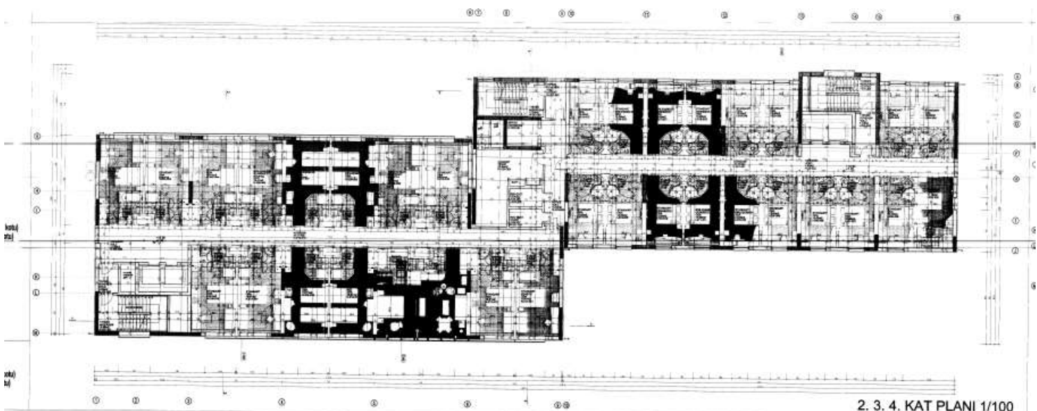
2. 3. 4. KAT PLANI 1/100
